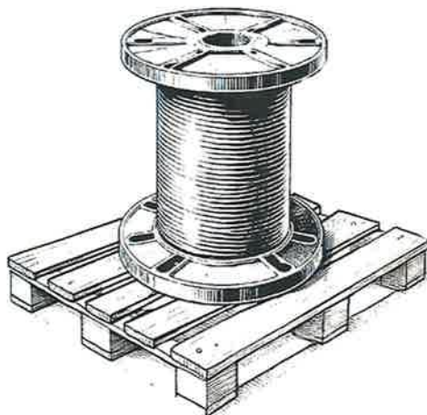
Rys. Bęben prawidłowo umieszczony na paletce do transportu samochodem ciężarowym.
